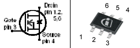
PG-SOT363
