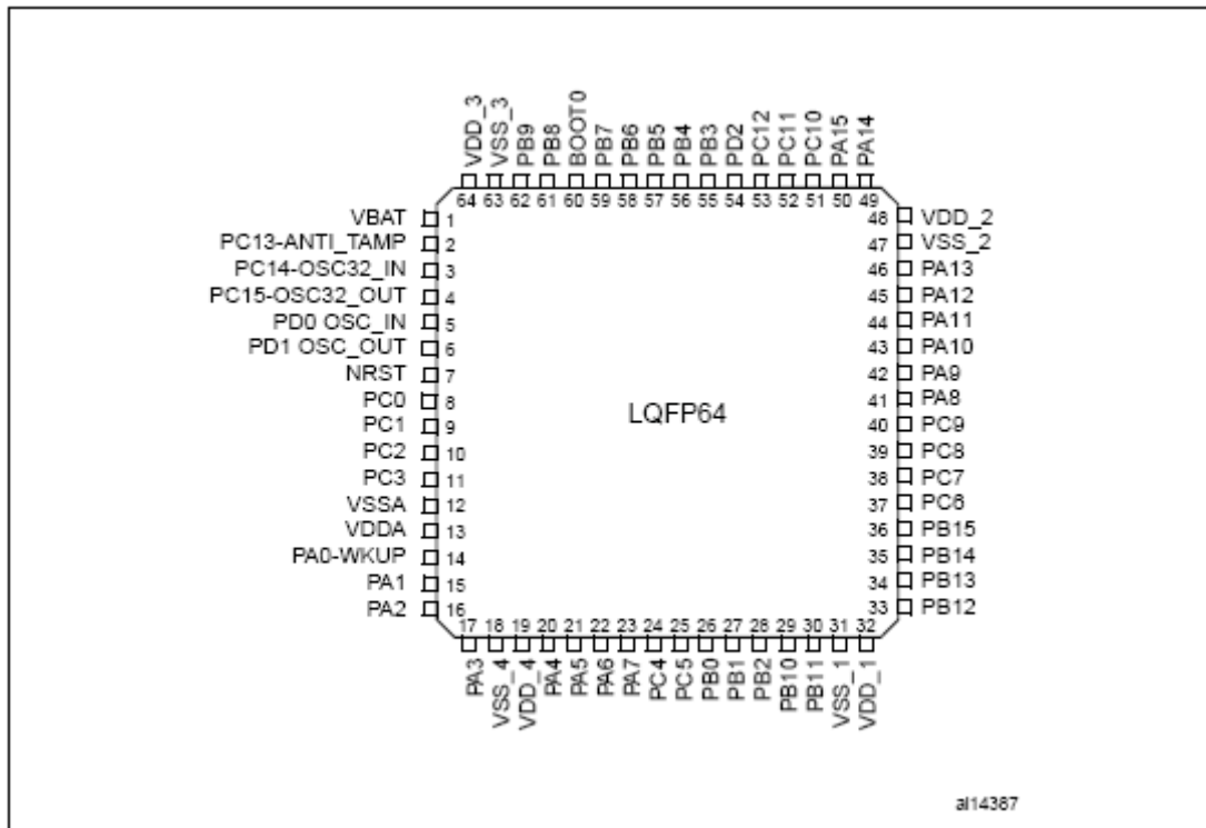
图4 STM32F101基本型LQFP64管脚
